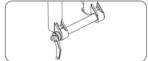
Steckachse in den Gabelausfallenden, ohne Nabe, Rock Shox® Abteil
